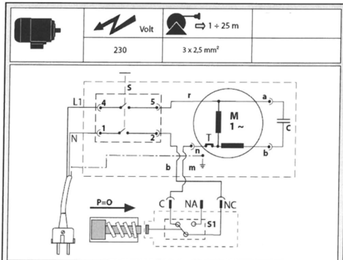
SCHEMA ELETTRICO / ELECTRICAL SCHEME
