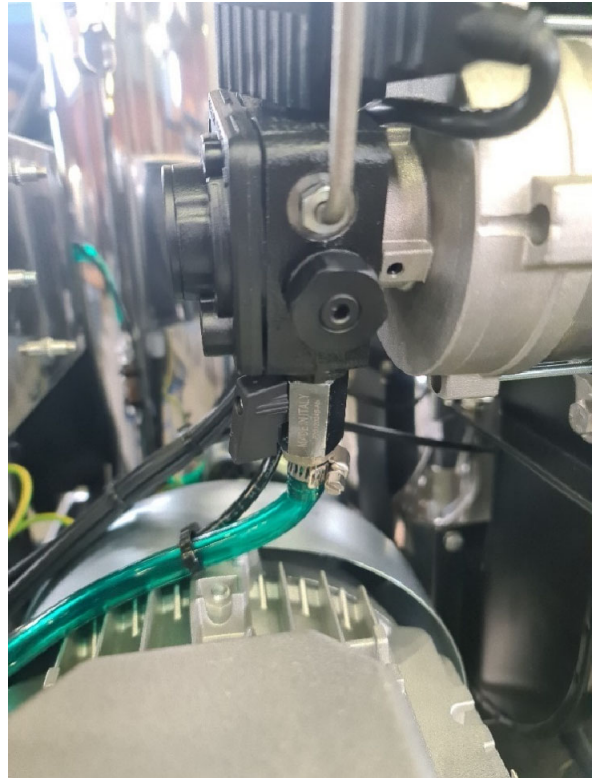
Válvula de bola para interrupción del suministro de gasóleo
