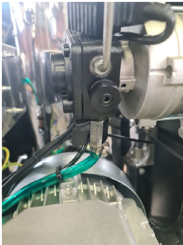
Válvula de bola para interrupción del suministro de gasóleo
